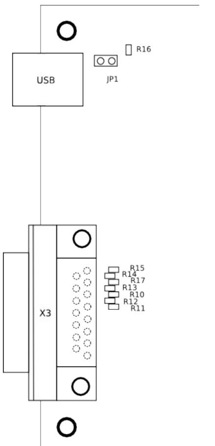
Abbildung 2: Konfiguration Master/Slave
