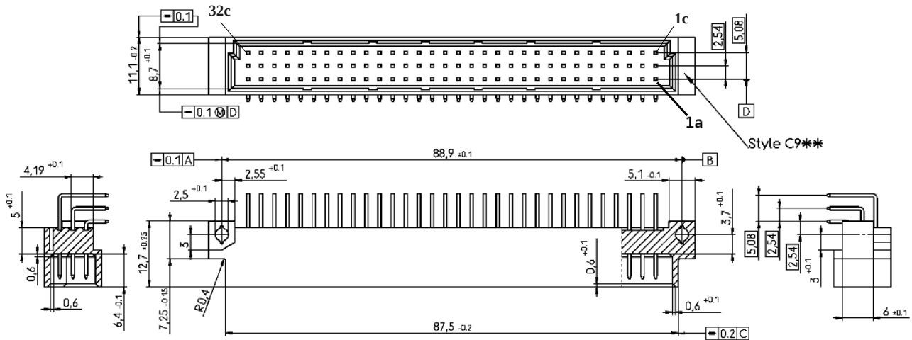
Abbildung 7: X1-Zeichnung
