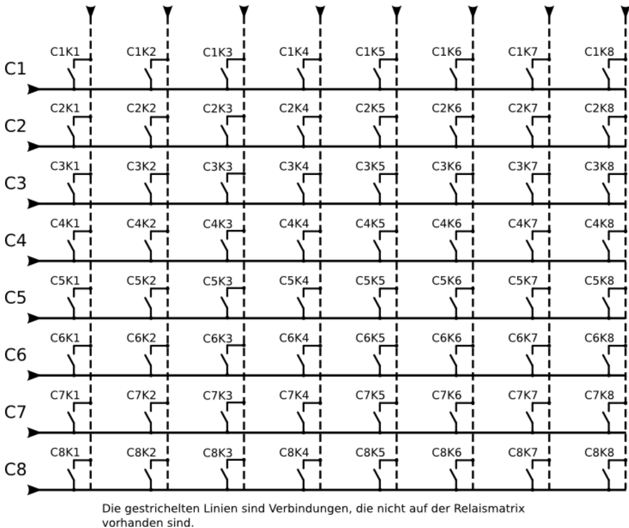
Abbildung 1: Kontaktplan
